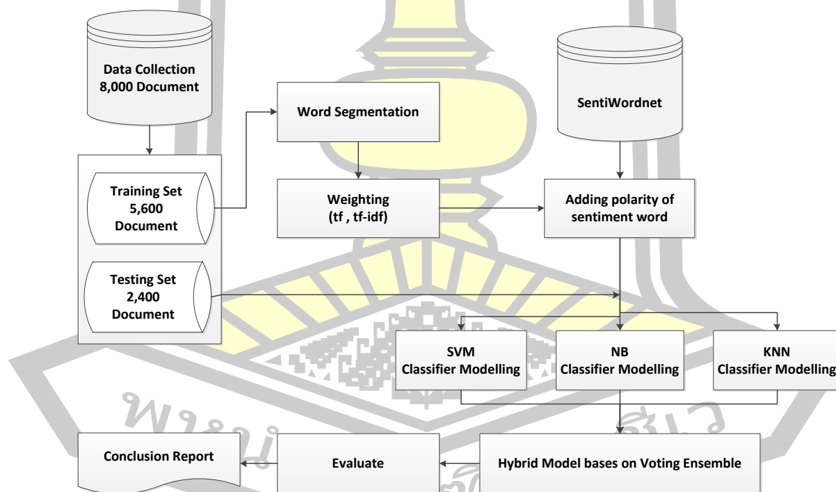
รูปที่ 3-3 แสดงกระบวนการดำเนินการวิจัย
