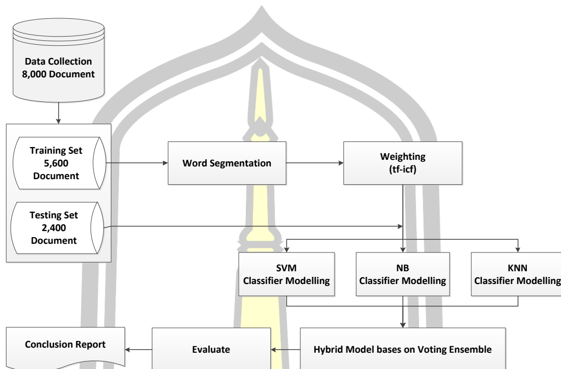
รูปที่ 3-7 กระบวนการดำเนินงานวิจัยที่ปรับปรุง
