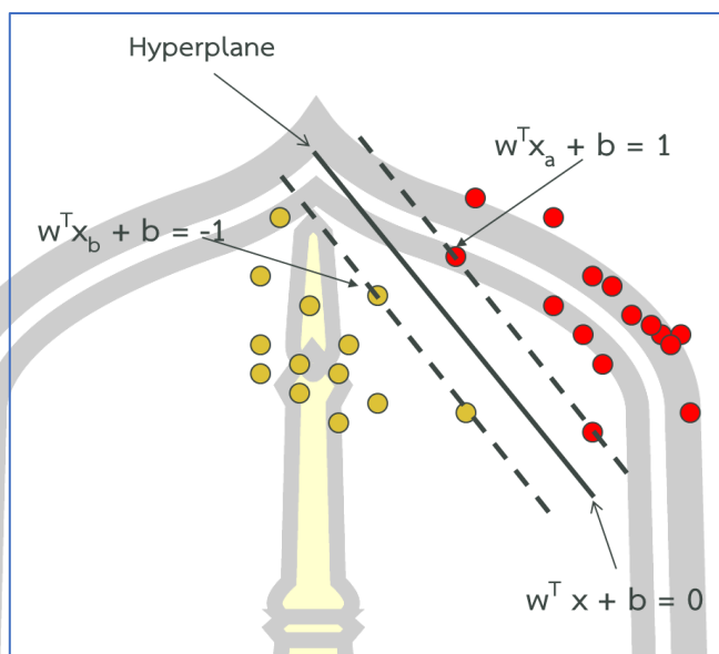
รูปที่ 2-7 ตัวอย่างการแบ่งกลุ่มข้อมูลโดยซัพพอร์ตเวกเตอร์แมชชีน
