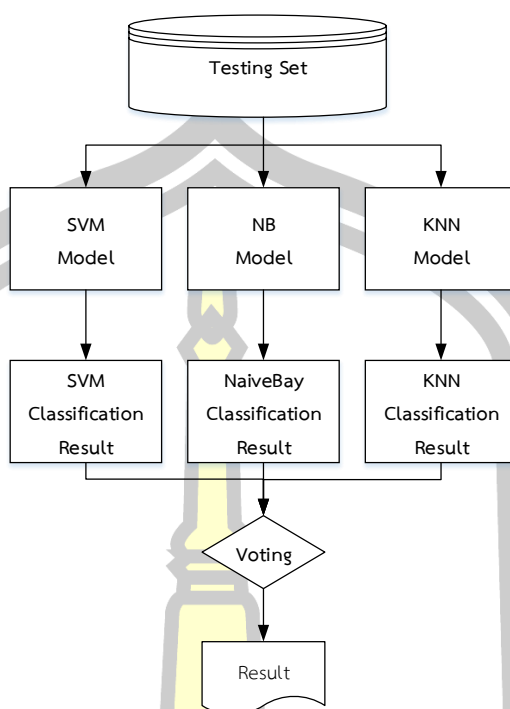
รูปที่ 3-6 การนำ Voting Ensemble Model มาใช้งาน
