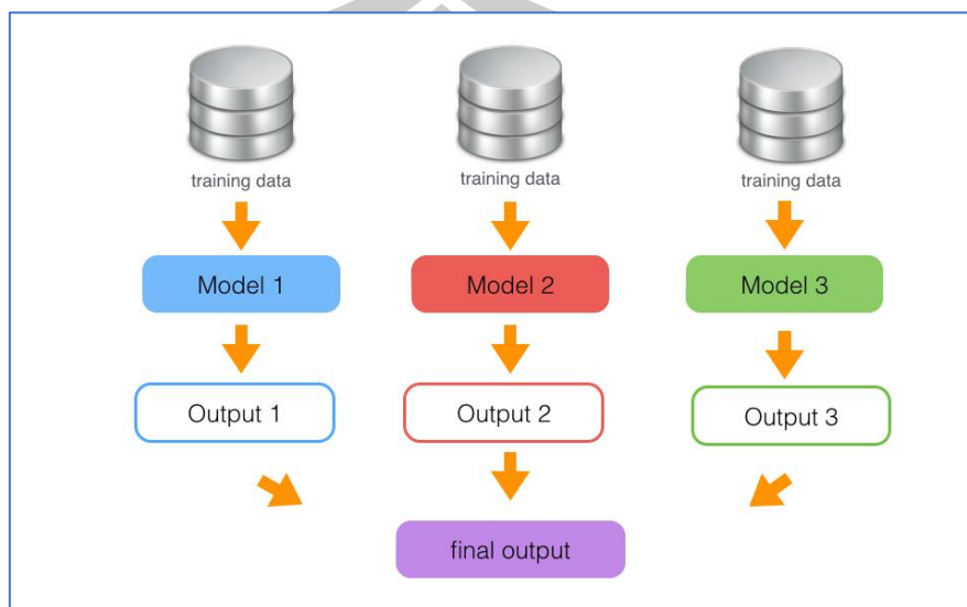
รูปที่ 2-9 แสดง concept การทำงานของ ensemble model
