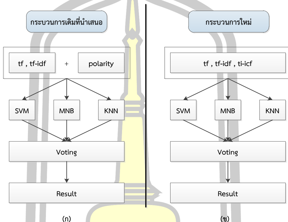
รูปที่ 4-2 แสดงการเปรียบเทียบกระบวนการในการสร้างโมเดลแบบเดิมและแบบใหม่
