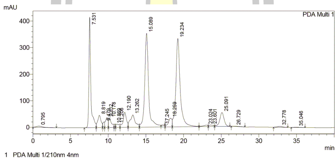
ภาพประกอบ 24 โครมาโตแกรมของ soluble oxalate ในตัวอย่างหน่อไม้ดิบ วิเคราะห์โดยใช้ HPLC
