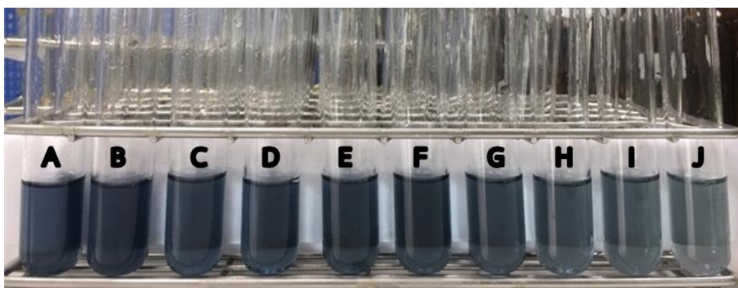
ภาพประกอบ 27 ผลการทดสอบ total phenolic contents ในตัวอย่างหน่อไม้บงหวาน
