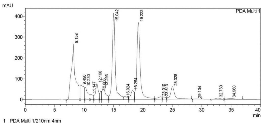
ภาพประกอบ 23 โครมาโตแกรมของ total oxalate ในตัวอย่างหน่อไม้ดิบ วิเคราะห์โดยใช้ HPLC
