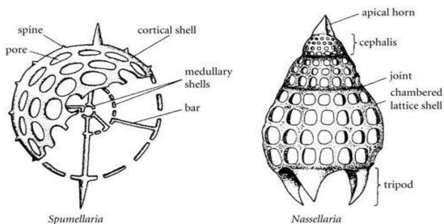
ภาพที่ 2 แสดงลักษณะพื้นฐานของกลุ่ม Spumellarian (ซ้าย) และกลุ่ม Nassellaria (ขวา) ดัดแปลงจาก: (Benton & Harper, 2009)
