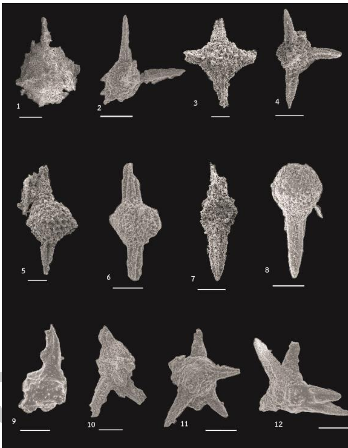
ภาพที่ 17 ภาพถ่าย Scanning Electron Microscope (SEM) ของเรดิโอลาเรียยุคดีโวเนียนจากพื้นที่หน้าตัดชั้นหินเชิร์ต บ้านวังผา อำเภopakหม จังหวัดเลย
