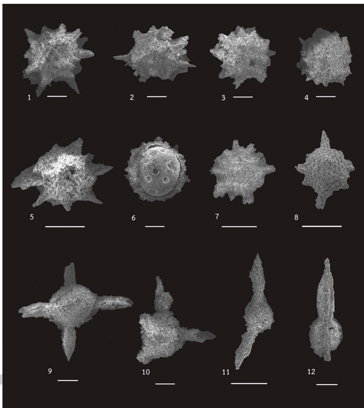
ภาพที่ 28 ภาพถ่าย Scanning Electron Microscope (SEM) ของเรดิโอลาเรียยุคดีโวเนียนจากพื้นที่หน้าตัดชั้นหินเชิร์ตบ้านกลาง อำเภอปากชม จังหวัดเลย
