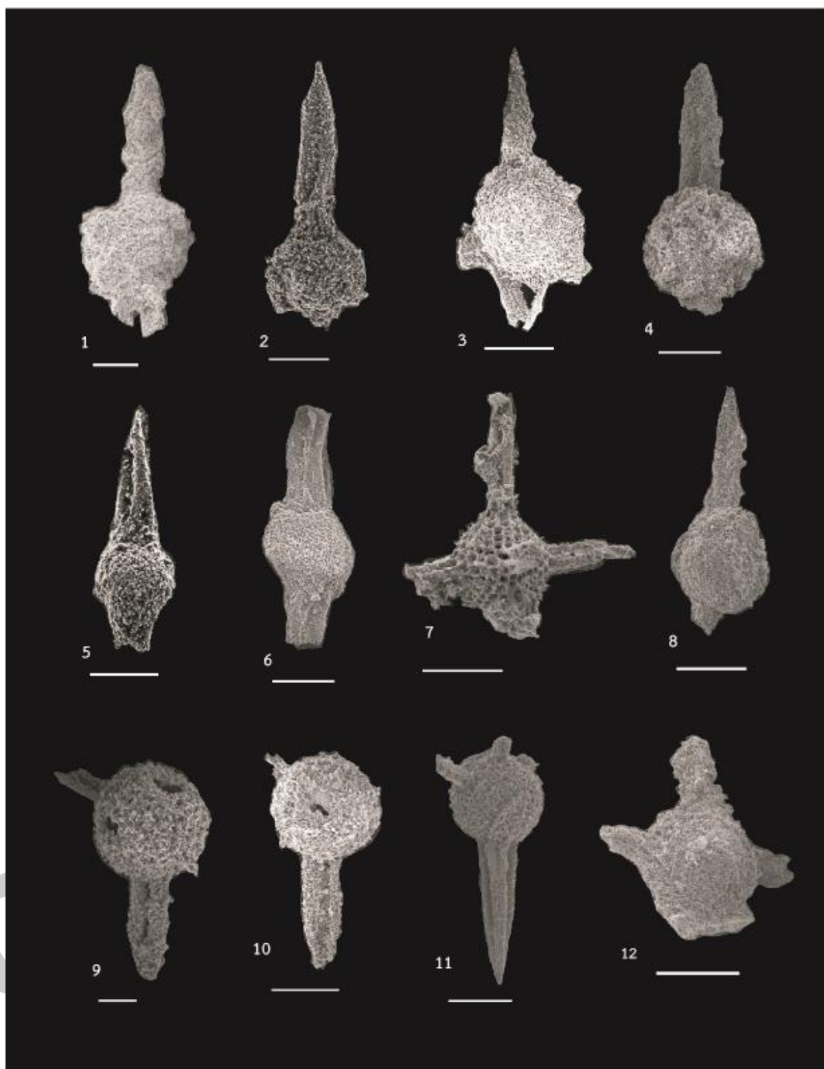
ภาพที่ 14 ภาพถ่าย Scanning Electron Microscope (SEM) ของเรดิโอลาเรียยุคทีโวเนียนจากพื้นที่หน้าตัดชั้นหินเชิร์ต บ้านวังผา อำเภopakชม จังหวัดเลย
