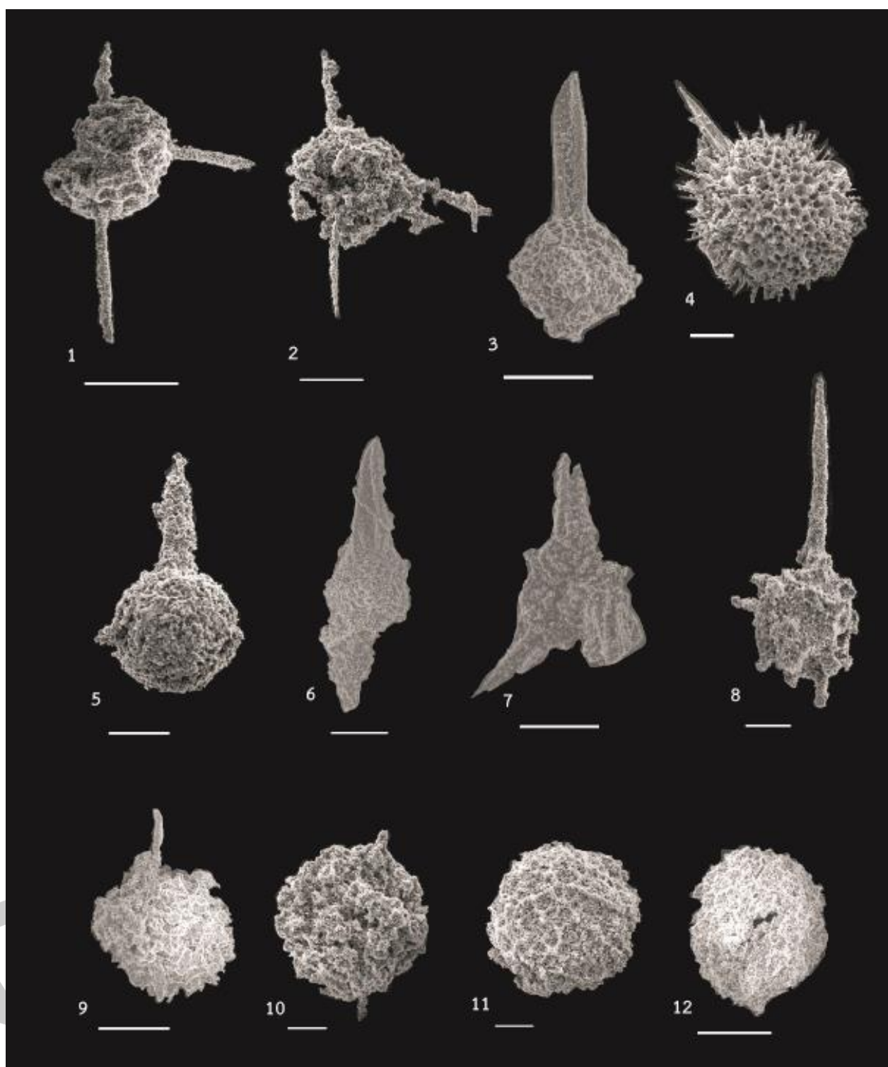
ภาพที่ 18 ภาพถ่าย Scanning Electron Microscope (SEM) ของเรดิโอลาเรียยุคดีโวเนียนจากพื้นที่หน้าตัดชั้นหินเชิร์ต บ้านวังผา อำเภอปากชม จังหวัดเลย
