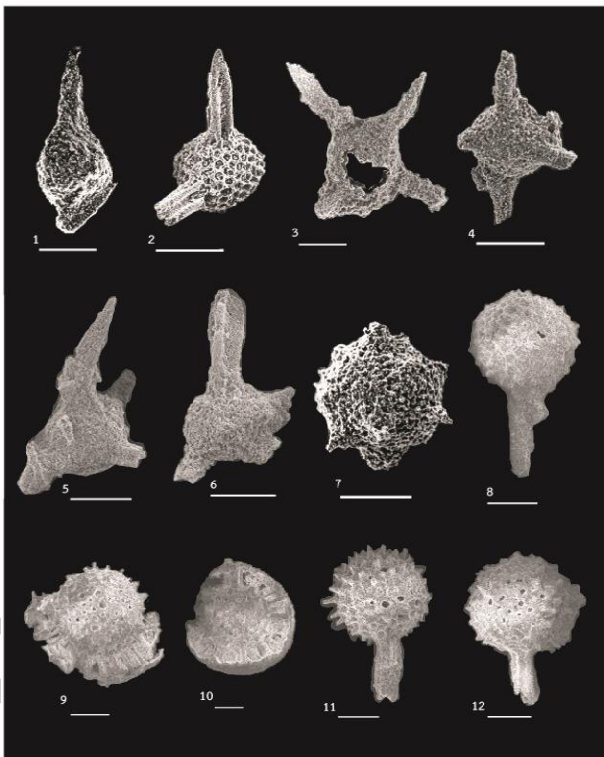
ภาพที่ 13 ภาพถ่าย Scanning Electron Microscope (SEM) ของเรติโโอลาเรียยุคดีโวเนียนจากพื้นที่หน้าตัดชั้นหินเชิร์ต บ้านวังผา อำเภopakชม จังหวัดเลย
