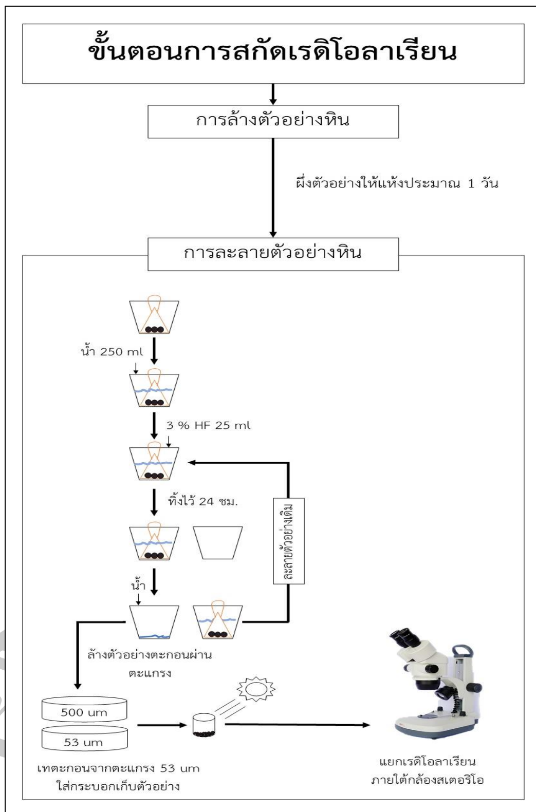
ภาพที่ 10 ภาพแผนผังแสดงขั้นตอนการสกัดเรติโอลาเรียนยุคดีโวเนียนจากหน้าตัดชั้นหินบ้านวังผา และบ้านกลาง อำเภopakชุม จังหวัดเลย
