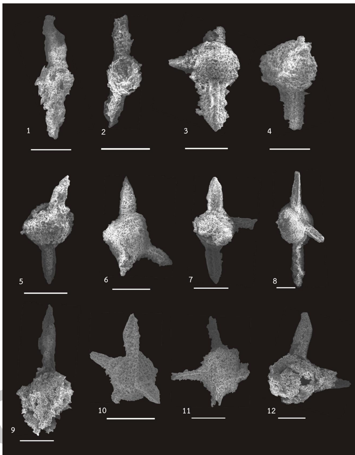
ภาพที่ 27 ภาพถ่าย Scanning Electron Microscope (SEM) ของเรดิโอลาเรียยุคไพลสโตซีนจากพื้นที่หน้าตัดชั้นหินเชิร์ตบ้านกลาง อำเภopakหม จังหวัดเลย
