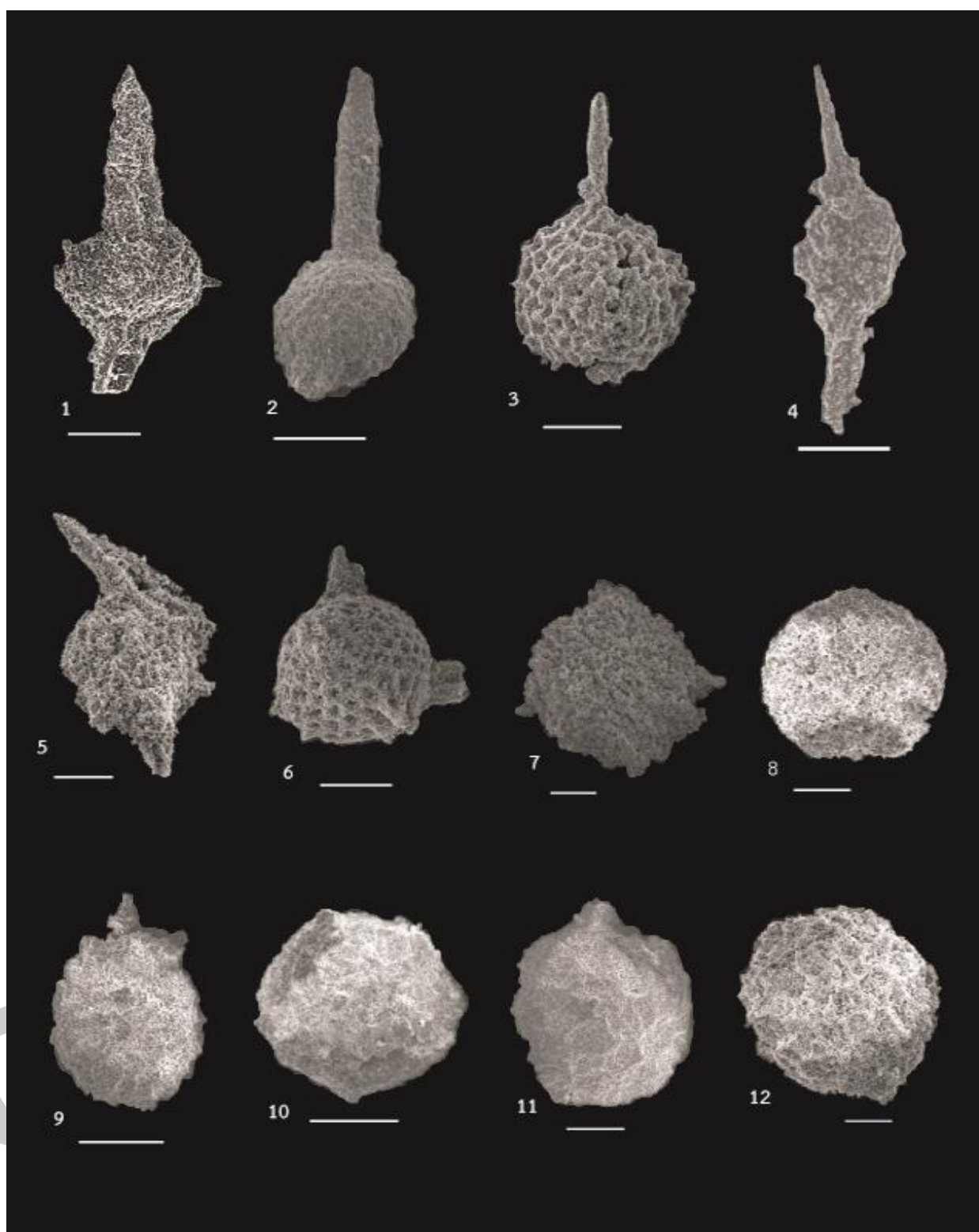
ภาพที่ 15 ภาพถ่าย Scanning Electron Microscope (SEM) ของเรดิโอลาเรียยุคทีโวเนียนจากพื้นที่หน้าตัดชั้นหินเชิร์ต บ้านวังผา อำเภopakชม จังหวัดเลย
