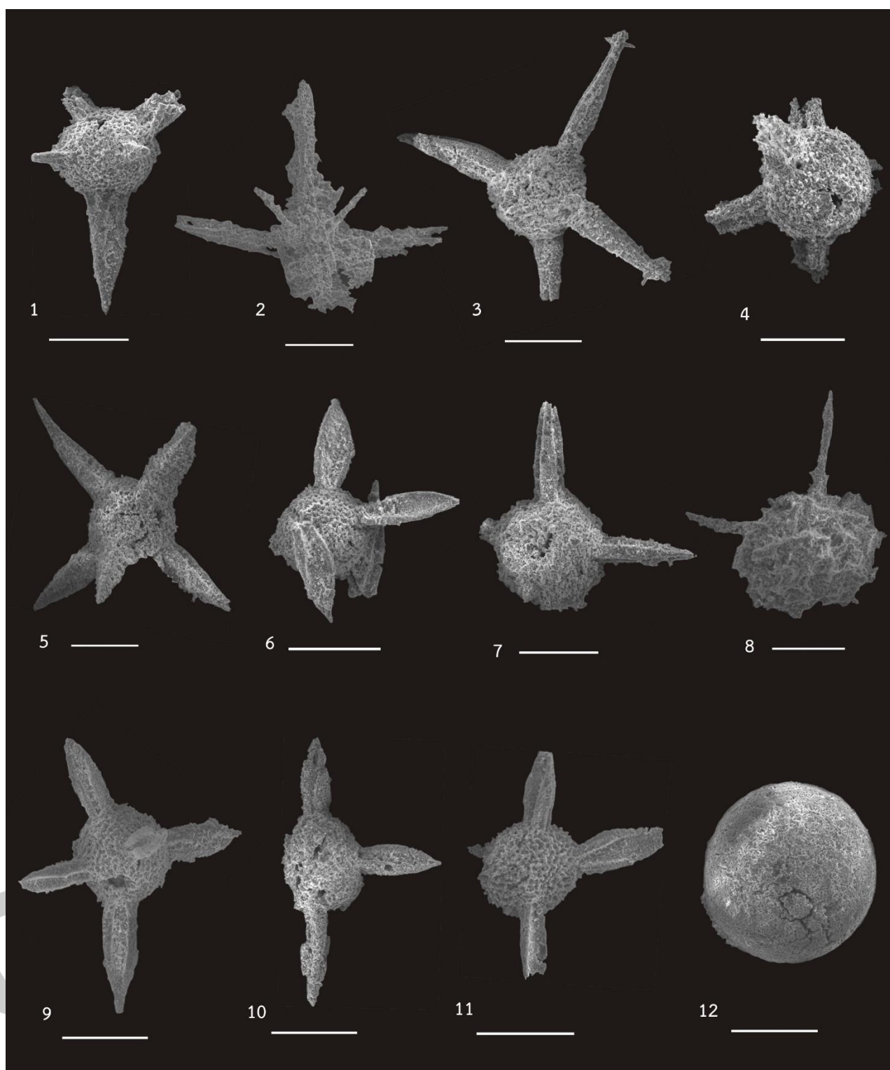
ภาพที่ 25 ภาพถ่าย Scanning Electron Microscope (SEM) ของเรดิโอลาเรียยุคทีโวเนียนจากพื้นที่หน้าตัดชั้นหินเชิร์ตบ้านกลาง อำเภopakหม จังหวัดเลย
