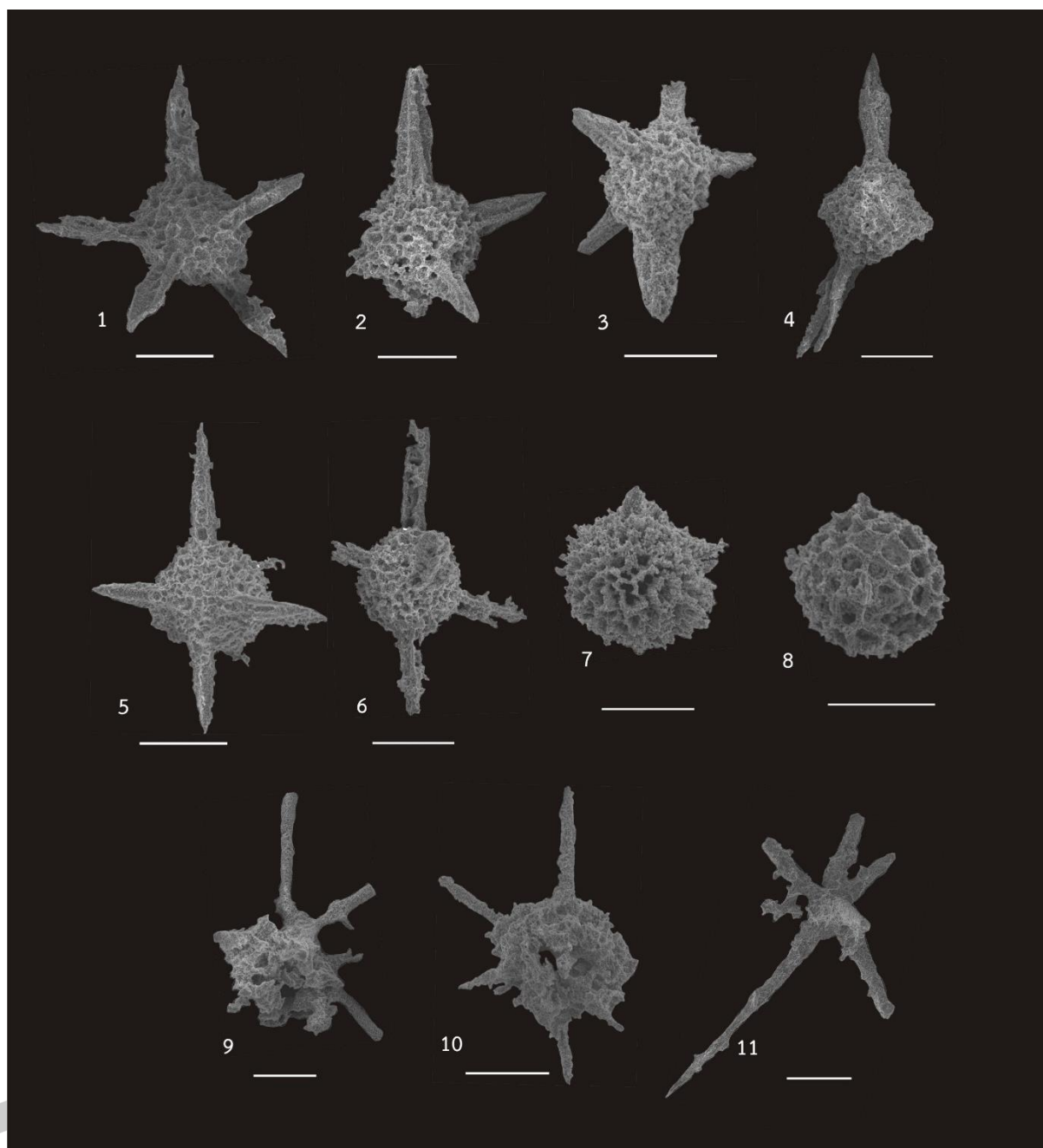
ภาพที่ 23 ภาพถ่าย Scanning Electron Microscope (SEM) ของเรดิโอลาเรียยุคดีโวเนียนจากพื้นที่หน้าตัดชั้นหินเขิร์ตบ้านวังผา อำเภopakหม จังหวัดเลย
