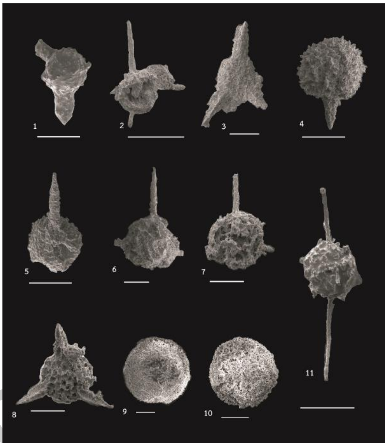
ภาพที่ 20 ภาพถ่าย Scanning Electron Microscope (SEM) ของเรดิโอลาเรียยุคทีโวเนียนจากพื้นที่หน้าตัดชั้นหินเชิร์ตบ้านวังผา อำเภอบางคนที จังหวัดเลย
