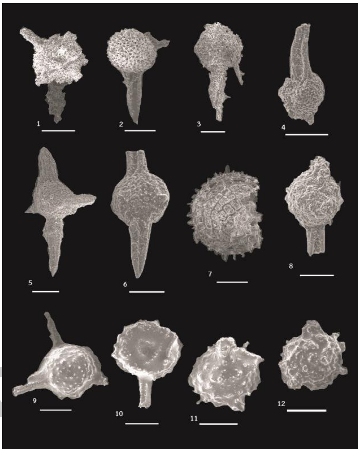
ภาพที่ 11 ภาพถ่าย Scanning Electron Microscope (SEM) ของเรติโอลาเรียยุคทีโวเนียนจากพื้นที่หน้าตัดชั้นหินเชิร์ต บ้านวังผา อำเภopakชม จังหวัดเลย
