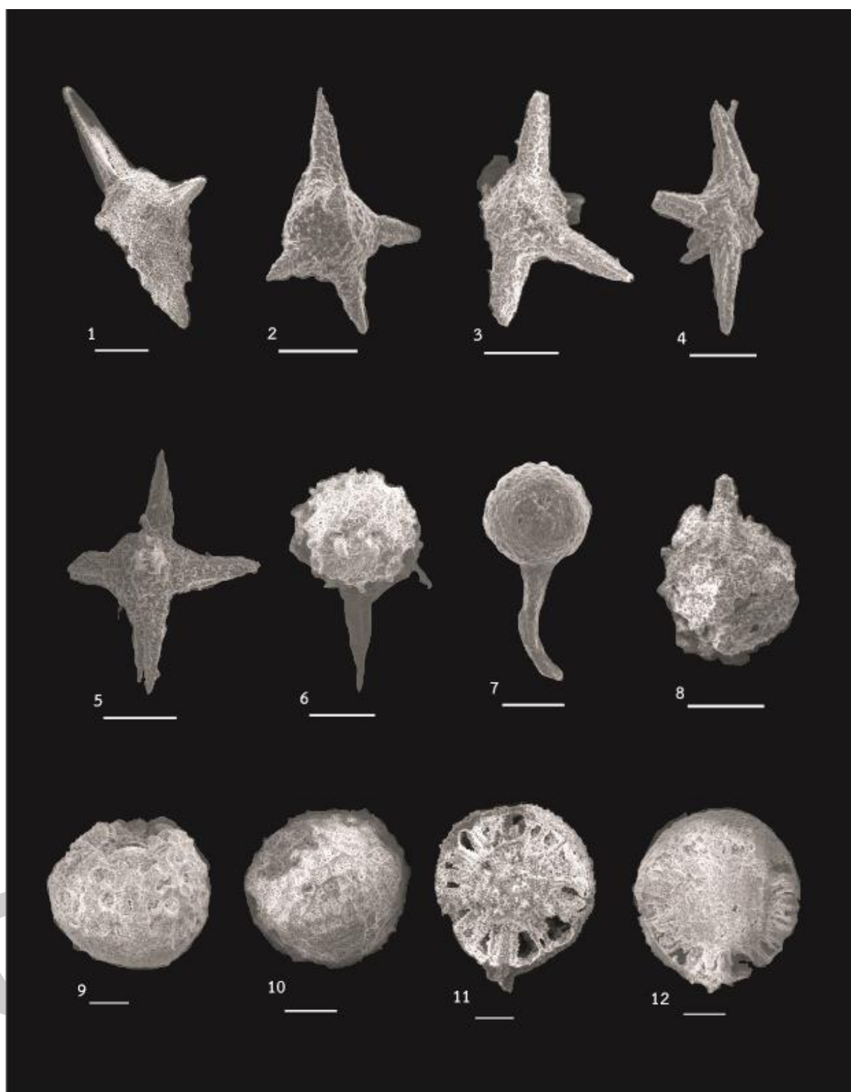
ภาพที่ 12 ภาพถ่าย Scanning Electron Microscope (SEM) ของเรดิโอลาเรียยุคทีโวเนียนจากพื้นที่หน้าตัดชั้นหินเชิร์ต บ้านวังผา อำเภอบางคนที จังหวัดเลย
