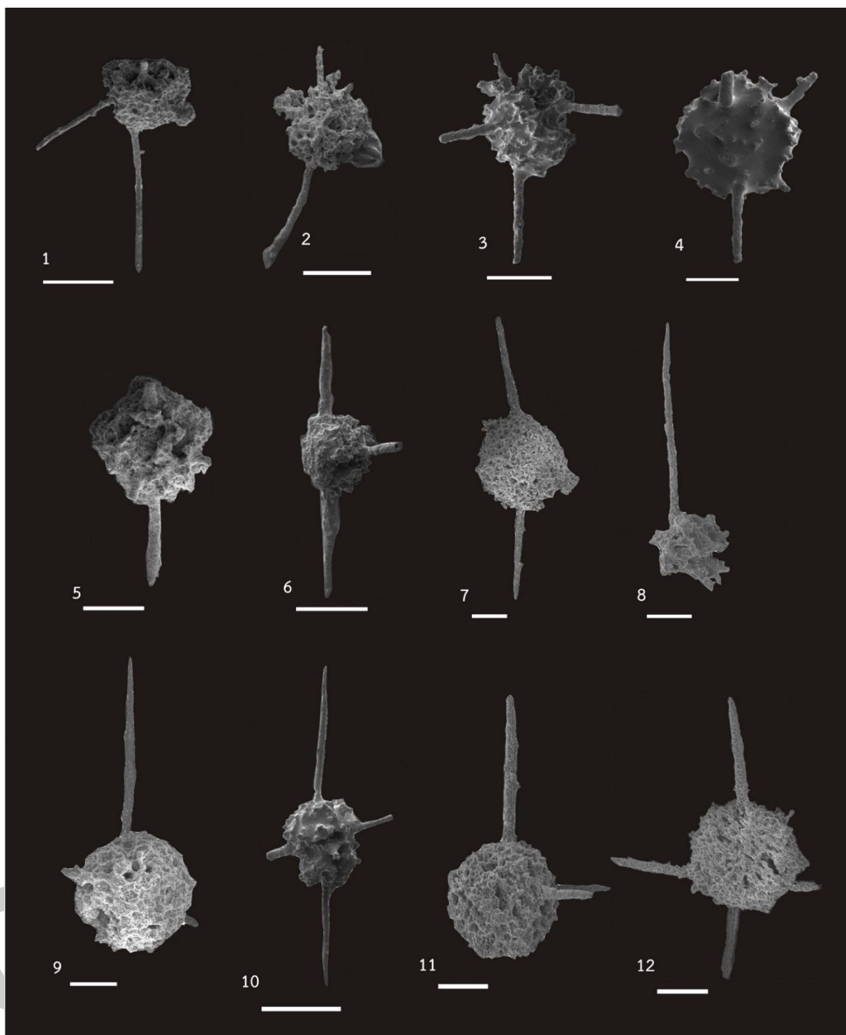
ภาพที่ 21 ภาพถ่าย Scanning Electron Microscope (SEM) ของเรดิโอลาเรียยุคดีโวเนียนจากพื้นที่หน้าตัดชั้นหินเชิร์ตบ้านวังผา อำเภopakชม จังหวัดเลย
