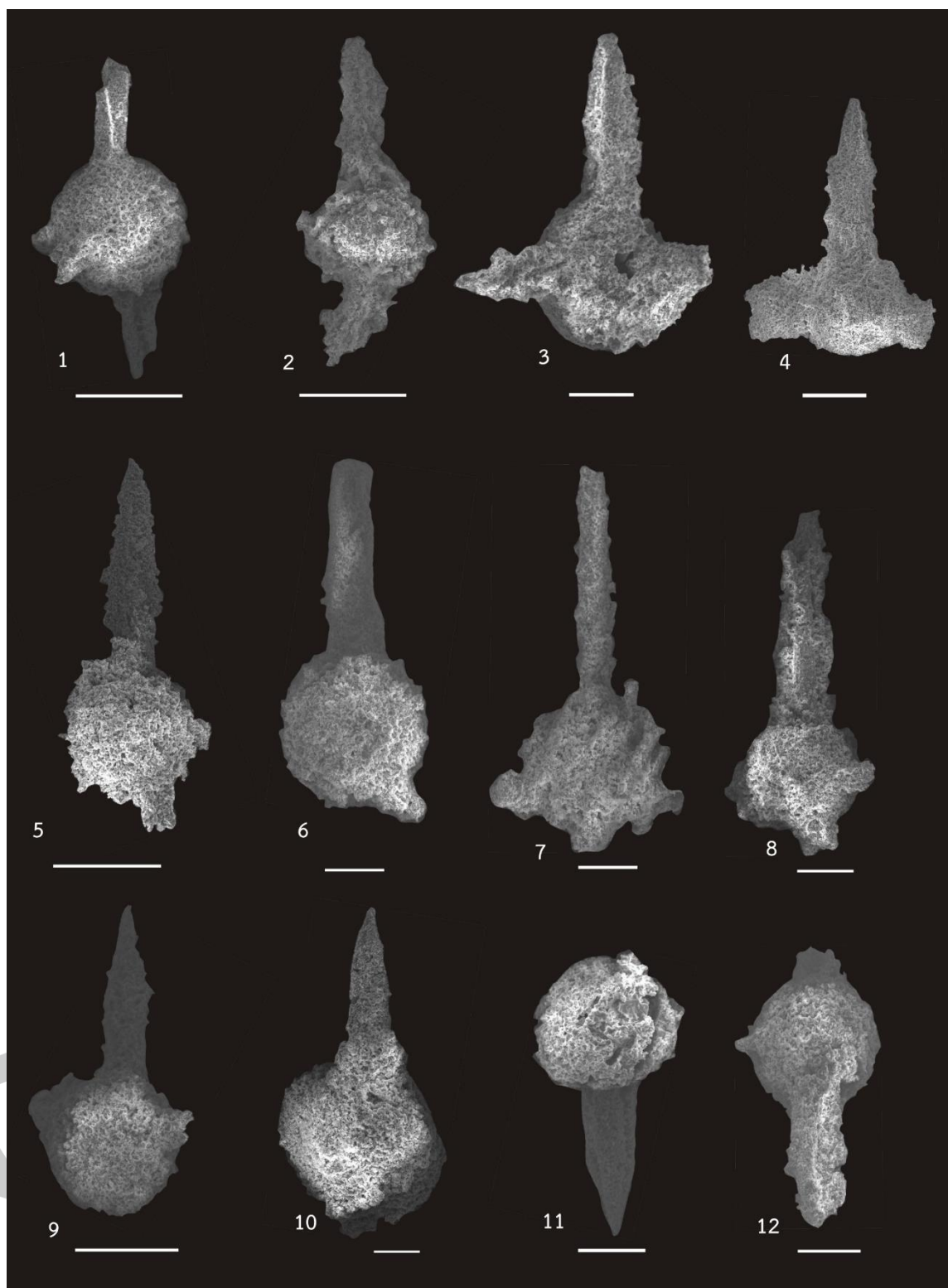
ภาพที่ 31 ภาพถ่าย Scanning Electron Microscope (SEM) ของเรติโอลาเรียยุคตีโวเนียนจากพื้นที่หน้าตัดชั้นหินเชิร์ตบ้านกลาง อำเภopakหม จังหวัดเลย
