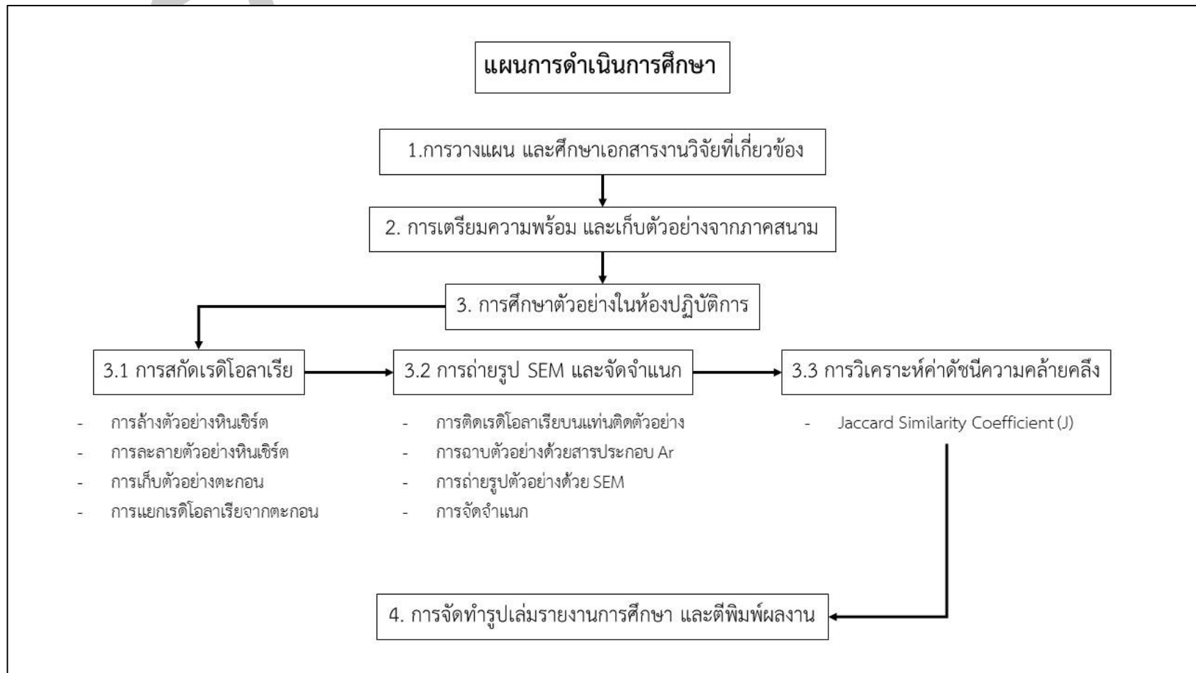
ภาพที่ 9 ภาพแผนผังแสดงขั้นตอนการดำเนินการศึกษาเรติโอลาเรียนยุคติวเนียนจากหน้าตัดชั้นหินบ้านวังผา และบ้านกลาง อำเภอปากชม จังหวัดเลย
