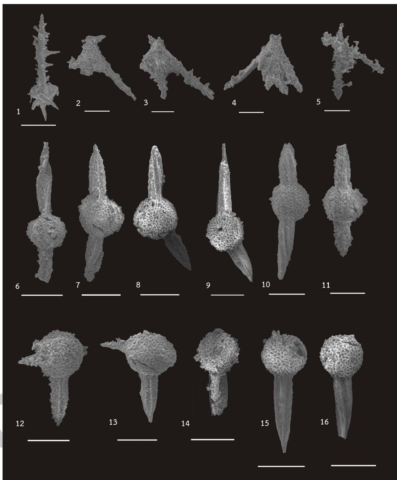
ภาพที่ 24 ภาพถ่าย Scanning Electron Microscope (SEM) ของเรดิโอลาเรียยุคดีโวเนียนจากพื้นที่หน้าตัดชั้นหินเชิร์ตบ้านกลาง อำเภopakหม จังหวัดเลย
