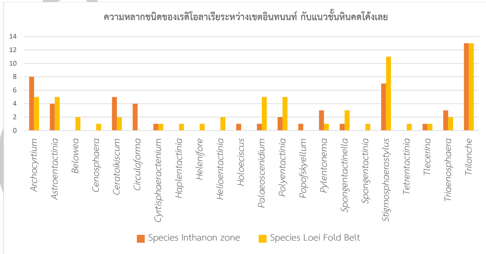
ภาพที่ 33 ภาพแสดงแผนภูมิการเทียบความหลากหลายของเรดิโอลาเรียนระหว่างเขตอินทนนท์ และแนวชั้นหินคดโค้งเลย
