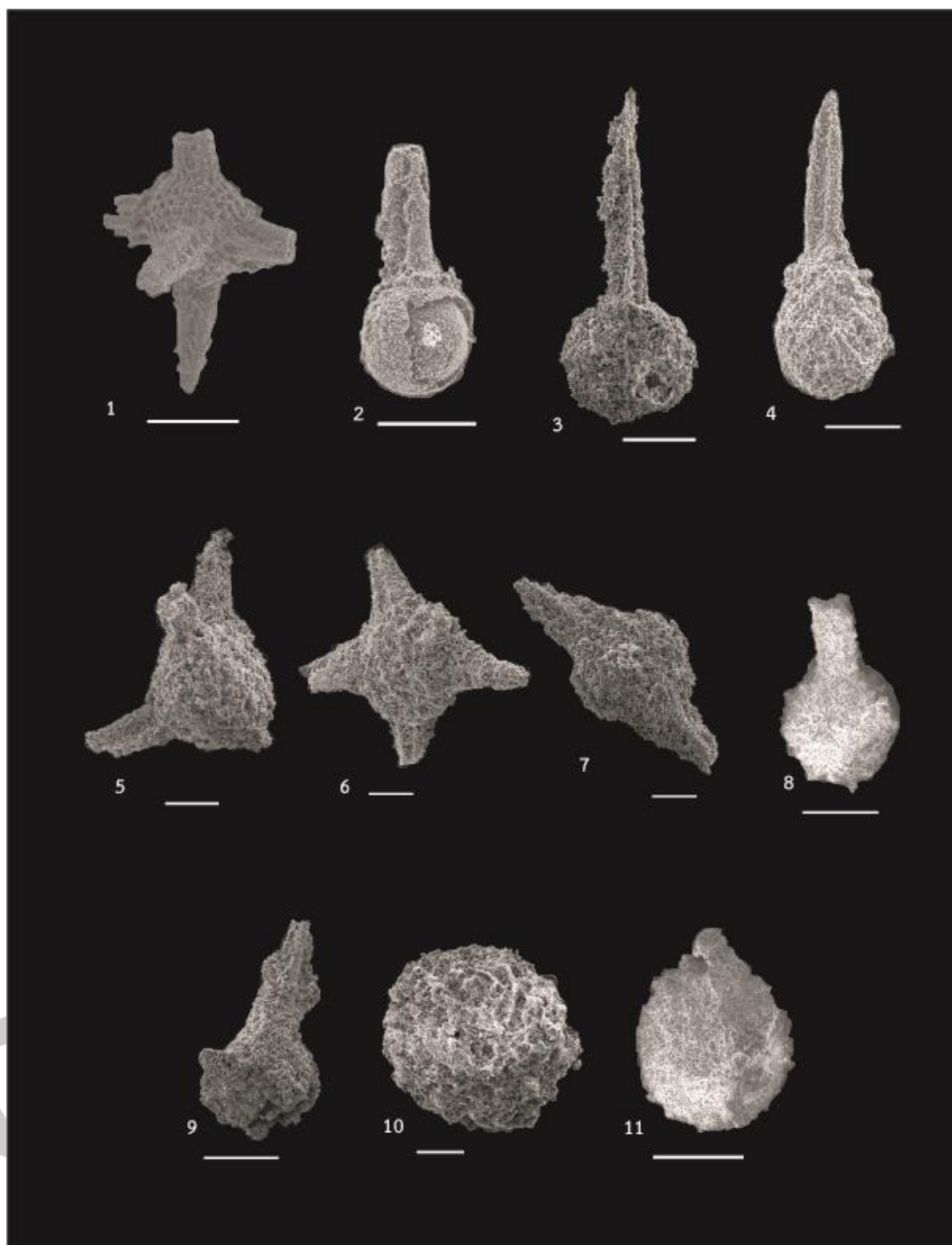
ภาพที่ 16 ภาพถ่าย Scanning Electron Microscope (SEM) ของเรติโอลาเรียยุคดีโวเนียนจากพื้นที่หน้าตัดชั้นหินเชิร์ต บ้านวังผา อำเภอปากชม จังหวัดเลย
