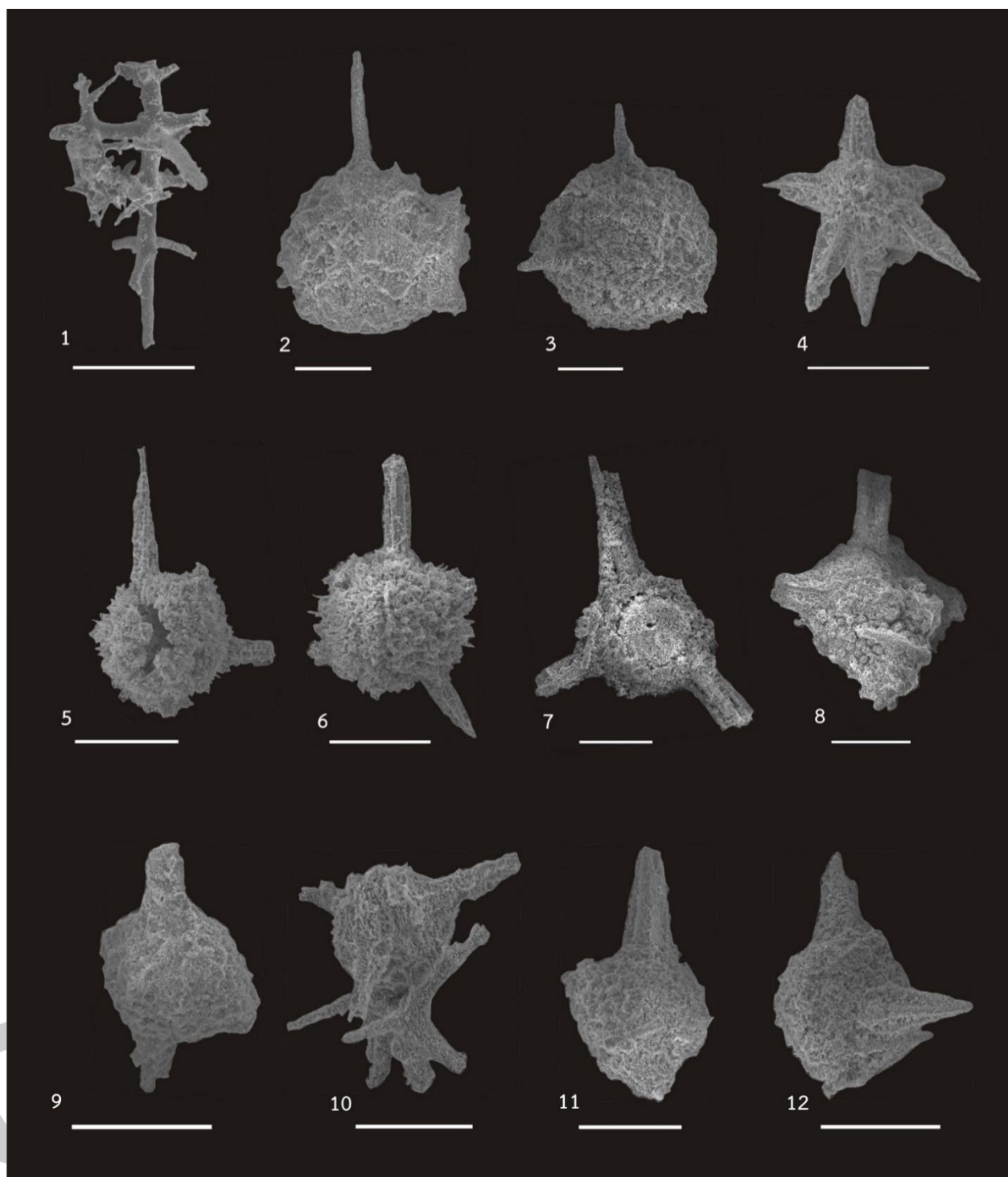
ภาพที่ 22 ภาพถ่าย Scanning Electron Microscope (SEM) ของเรดิโอลาเรียยุคติวเนียนจากพื้นที่หน้าตัดชั้นหินเชิร์ตบ้านวังผา อำเภอบางขัน จังหวัดเลย ภาคตะวันออกเฉียงเหนือของประเทศไทย
