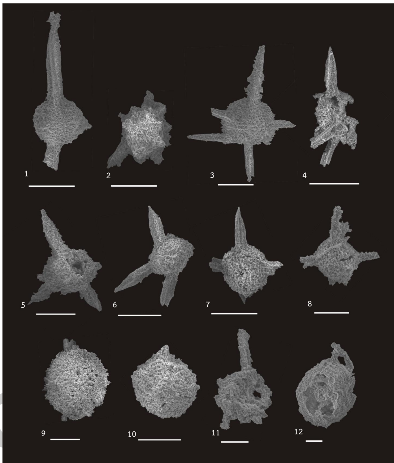
ภาพที่ 26 ภาพถ่าย Scanning Electron Microscope (SEM) ของเรดิโอลาเรียยุคทีโวเนียนจากพื้นที่หน้าตัดชั้นหินเชิร์ตบ้านกลาง อำเภopakหม จังหวัดเลย
