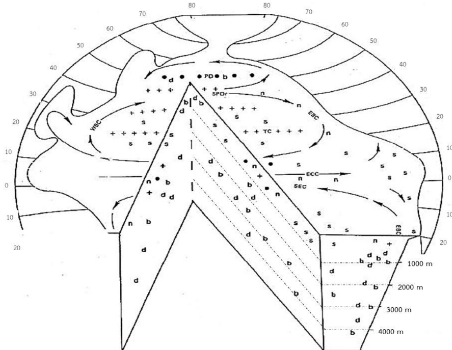
ภาพที่ 3 แสดงตำแหน่งการกระจายตัวของเรดิโอไลเรียนตามพฤติกรรมการกินโดยจะแบ่งออกเป็น 4 ประเภทหลักดังนี้ b: bacterivores, n: nannoherbivores หรือ herbivores, s: symbiotrophes, d: detritivores (ดัดแปลงจาก: (Casey, 1993))
