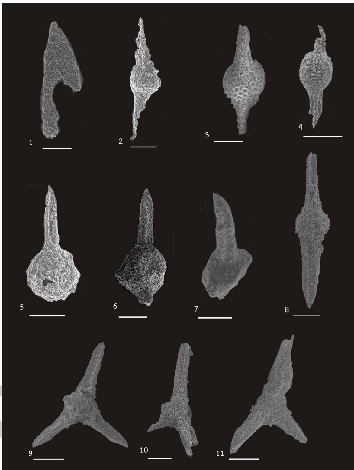
ภาพที่ 19 ภาพถ่าย Scanning Electron Microscope (SEM) ของเรติโปลาเรียยุคดีโวเนียนจากพื้นที่หน้าตัดชั้นหินเชิร์ตบ้านวังผา อำเภopakชม จังหวัดเลย
