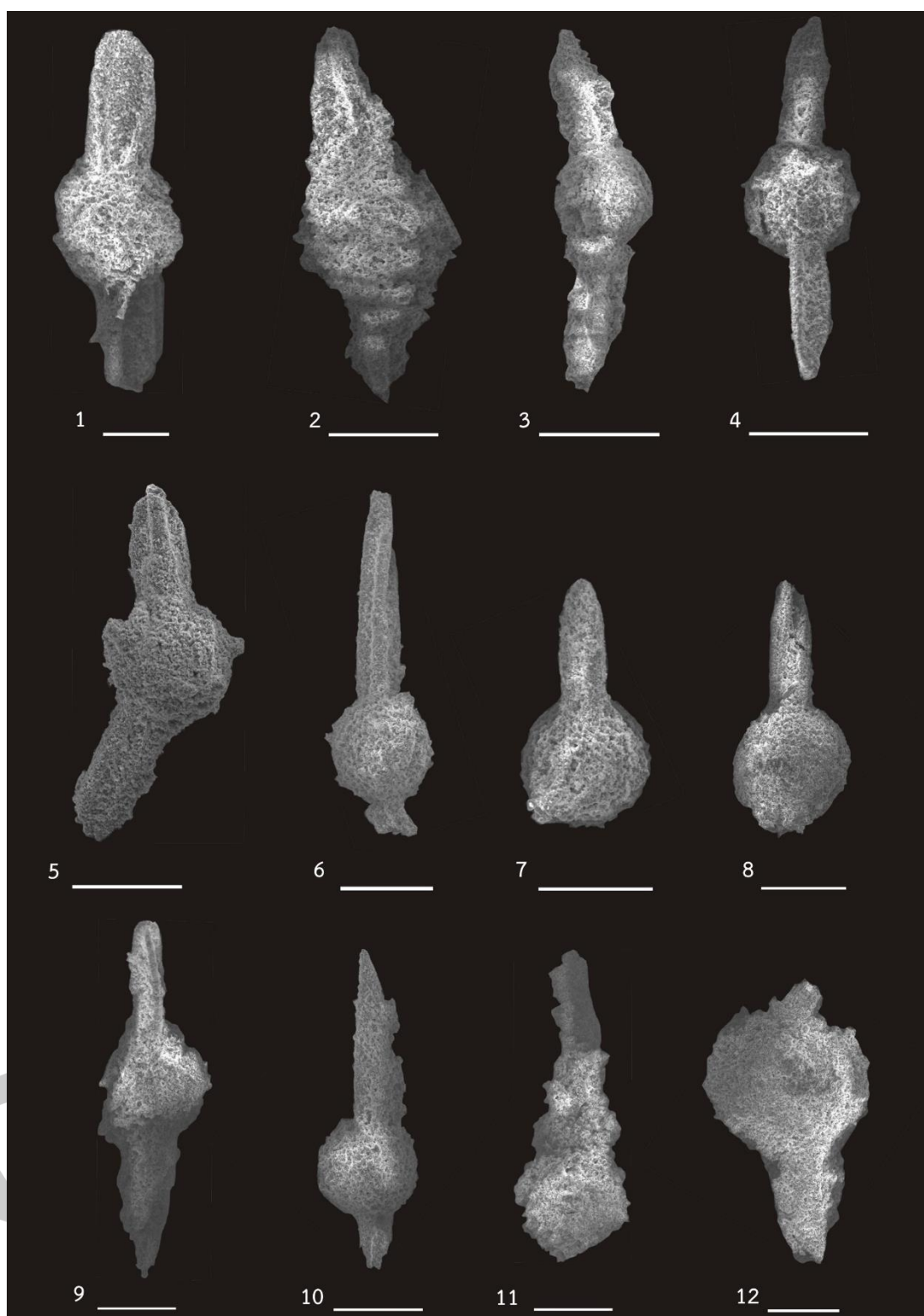
ภาพที่ 29 ภาพถ่าย Scanning Electron Microscope (SEM) ของเรดิโอลาเรียยุคทีโวเนียนจากพื้นที่หน้าตัดชั้นหินเชิร์ตบ้านกลาง อำเภopakหม จังหวัดเลย
