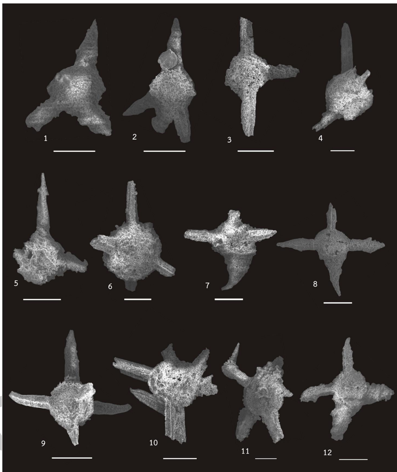
ภาพที่ 30 ภาพถ่าย Scanning Electron Microscope (SEM) ของเรดิโอลาเรียยุคทีโอเนียนจากพื้นที่หน้าตัดชั้นหินเชิร์ตบ้านกลาง อำเภopakหม จังหวัดเลย
