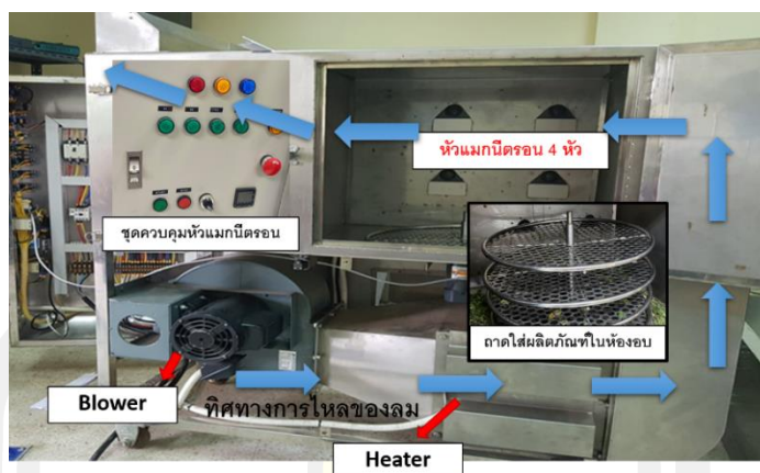
ภาพประกอบ 10 แผนผังโครงสร้างเครื่องอบแห้งไมโครเวฟร่วมกับลมร้อน
