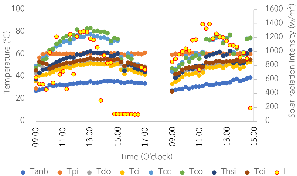
ภาพประกอบ ข-5 ความสัมพันธ์ระหว่างอุณหภูมิตัวกลางที่จุดต่าง ๆ กับเวลาเมื่ออบแห้งที่ 60 °C กำลังอินฟราเรด 1,000 W
