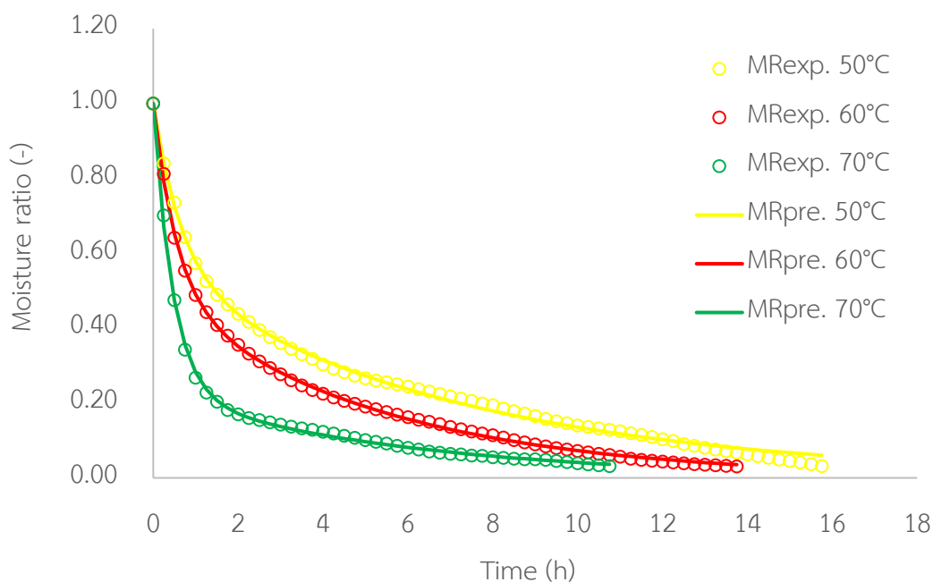
ภาพประกอบ 4.6 การเปลี่ยนแปลงอัตราส่วนความชื้นจากผลการทำนายของสมการ Verma et. al. เปรียบเทียบกับการทดลองอบแห้งที่กำลังอินฟราเรด 1,000 W
