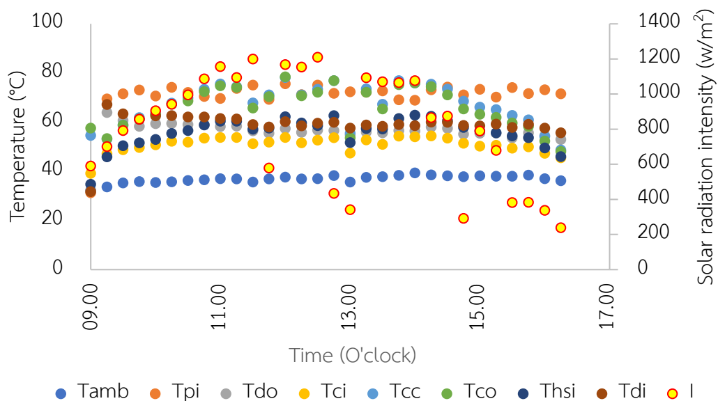
ภาพประกอบ ข-9 ความสัมพันธ์ระหว่างอุณหภูมิตัวกลางที่จุดต่าง ๆ กับเวลาเมื่ออบแห้งที่ 70 °C กำลังอินฟราเรด 1,500 W
