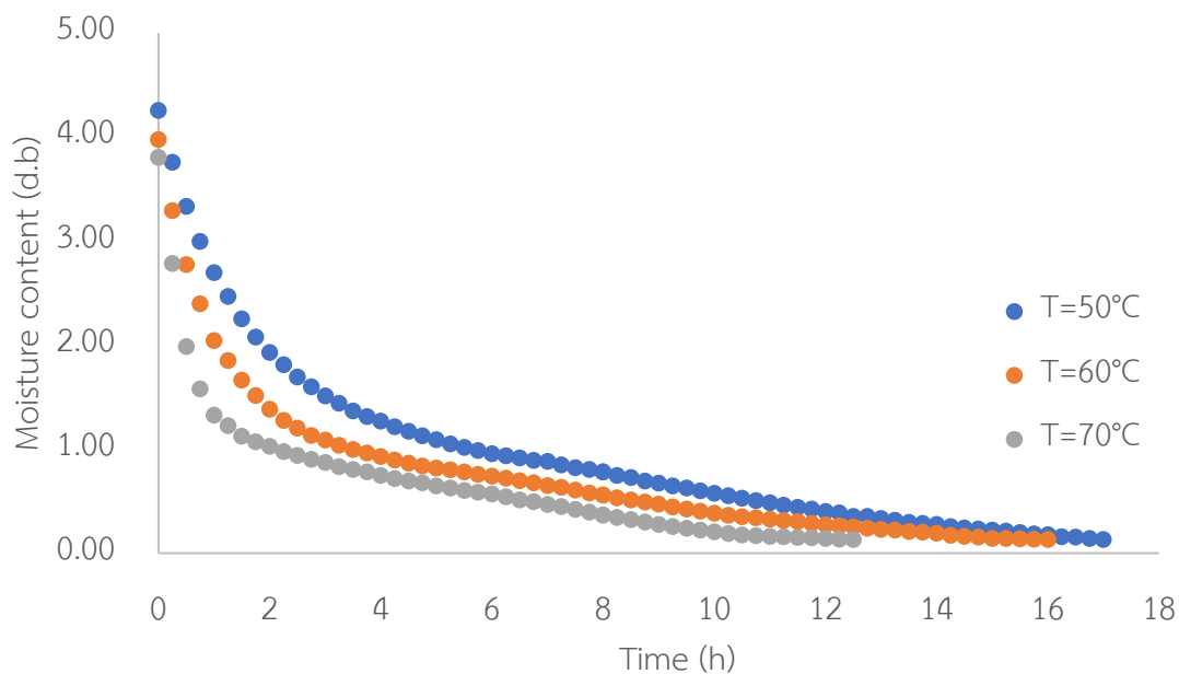
ภาพประกอบ 4.2 ความชื้นในแต่ละเวลาการอบแห้งโดยใช้กำลังอินฟราเรดขนาด 500 W อบแห้งที่อุณหภูมิภายในชั้นโพลแตกต่างกัน
