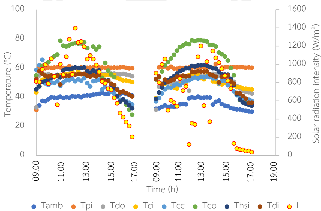
ภาพประกอบ ข-2 ความสัมพันธ์ระหว่างอุณหภูมิตัวกลางที่จุดต่าง ๆ กับเวลาเมื่ออบแห้งที่ 60 °C กำลังอินฟราเรด 500 W
