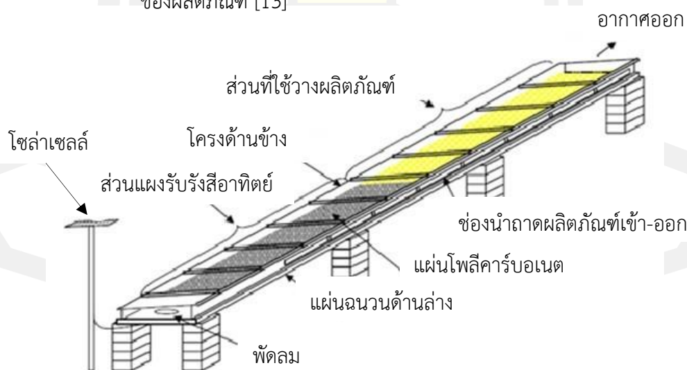
ภาพประกอบ 2.5 เครื่องอบแห้งแบบใช้แผงรับความร้อนโดยใช้พัดลมดูดอากาศร้อนเพื่อลดความชื้นของผลิตภัณฑ์ [13]
