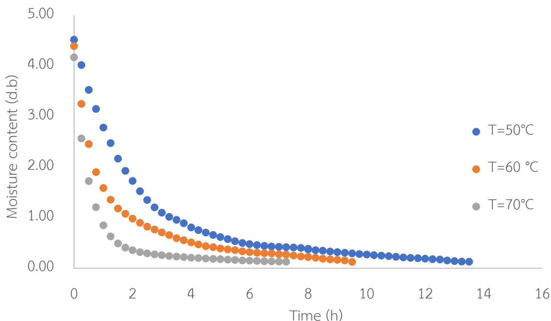
ภาพประกอบ 4.4 ความชื้นในแต่ละเวลาการอบแห้งโดยใช้กำลังอินฟราเรดขนาด 1,500 W อบแห้งที่อุณหภูมิภายในชิ้นโพลแตกต่างกัน
