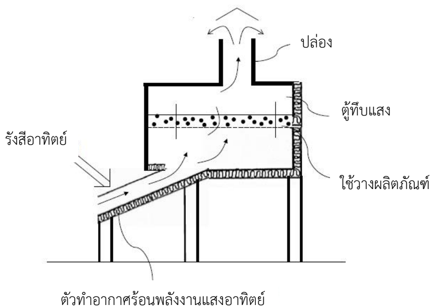
ภาพประกอบ 2.3 เครื่องอบแห้งแบบใช้แผงรับแสงอาทิตย์ [15]
