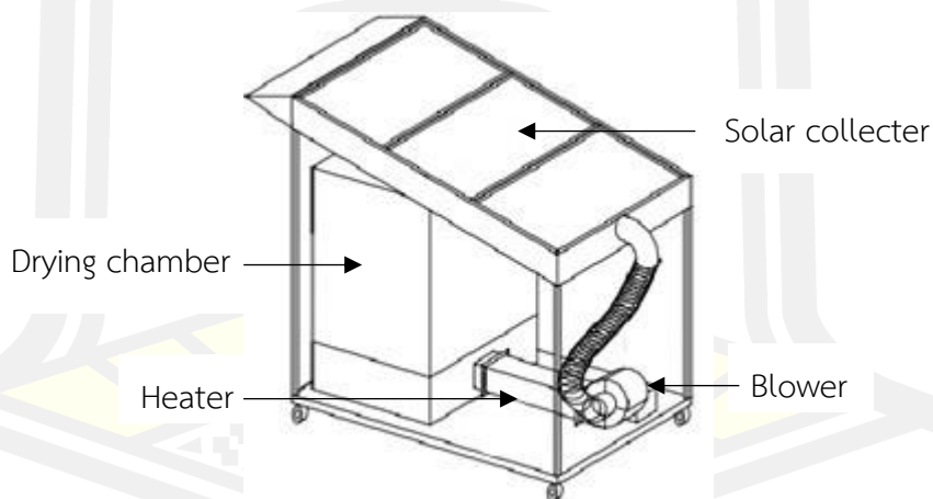
ภาพประกอบ 2.8 ตู้อบพลังงานแสงอาทิตย์ร่วมฮีตเตอร์ไฟฟ้า [13]
