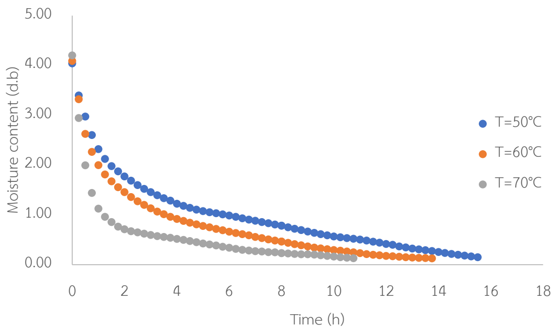
ภาพประกอบ 4.3 ความชื้นในแต่ละเวลาการอบแห้งโดยใช้กำลังอินฟราเรดขนาด 1,000 W อบแห้งที่อุณหภูมิภายในชั้นโพลแตกต่างกัน
