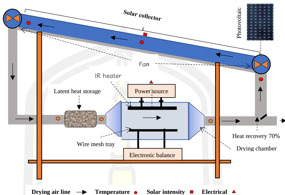
ภาพประกอบ 3.15 ตำแหน่งของการวัดอุณหภูมิ ความเข้มรังสีอาทิตย์ พลังงานไฟฟ้า และการซังมวลของไหล
