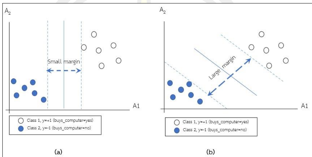
ภาพที่ 1 แสดง Hyperplanes ระหว่าง (a) ขอบขนาดเล็ก และ (b) ขอบขนาดใหญ่ (Han et al., 2012)
