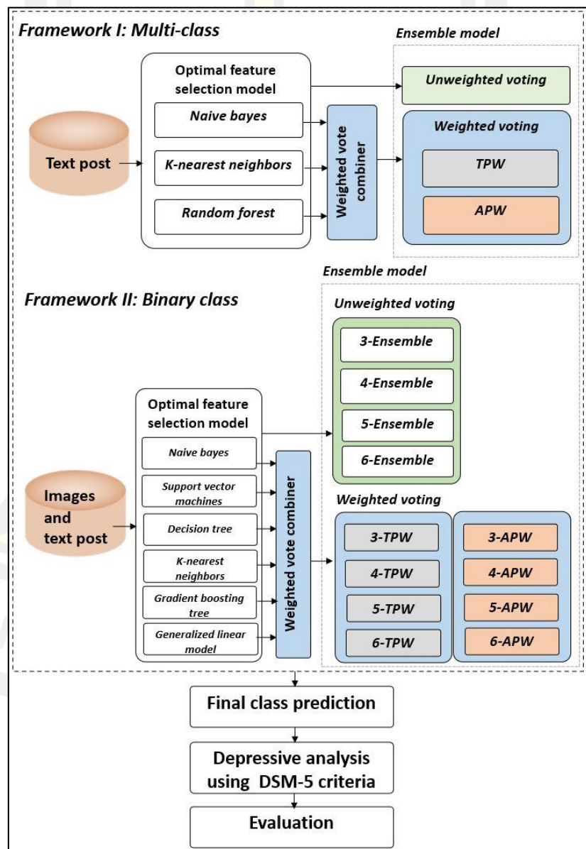
ภาพที่ 3 กรอบการวิจัยการปรับปรุงวิธีการการพยากรณ์โรคซึมเศร้าในวัยรุ่น
