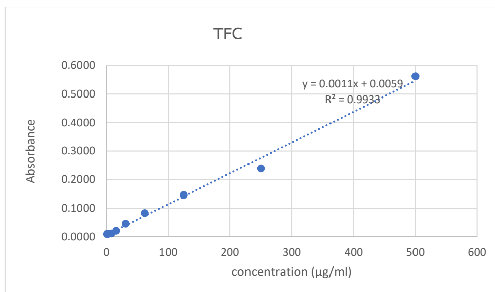
ภาพภาคผนวก 4 กราฟมาตรฐานของ TFC
