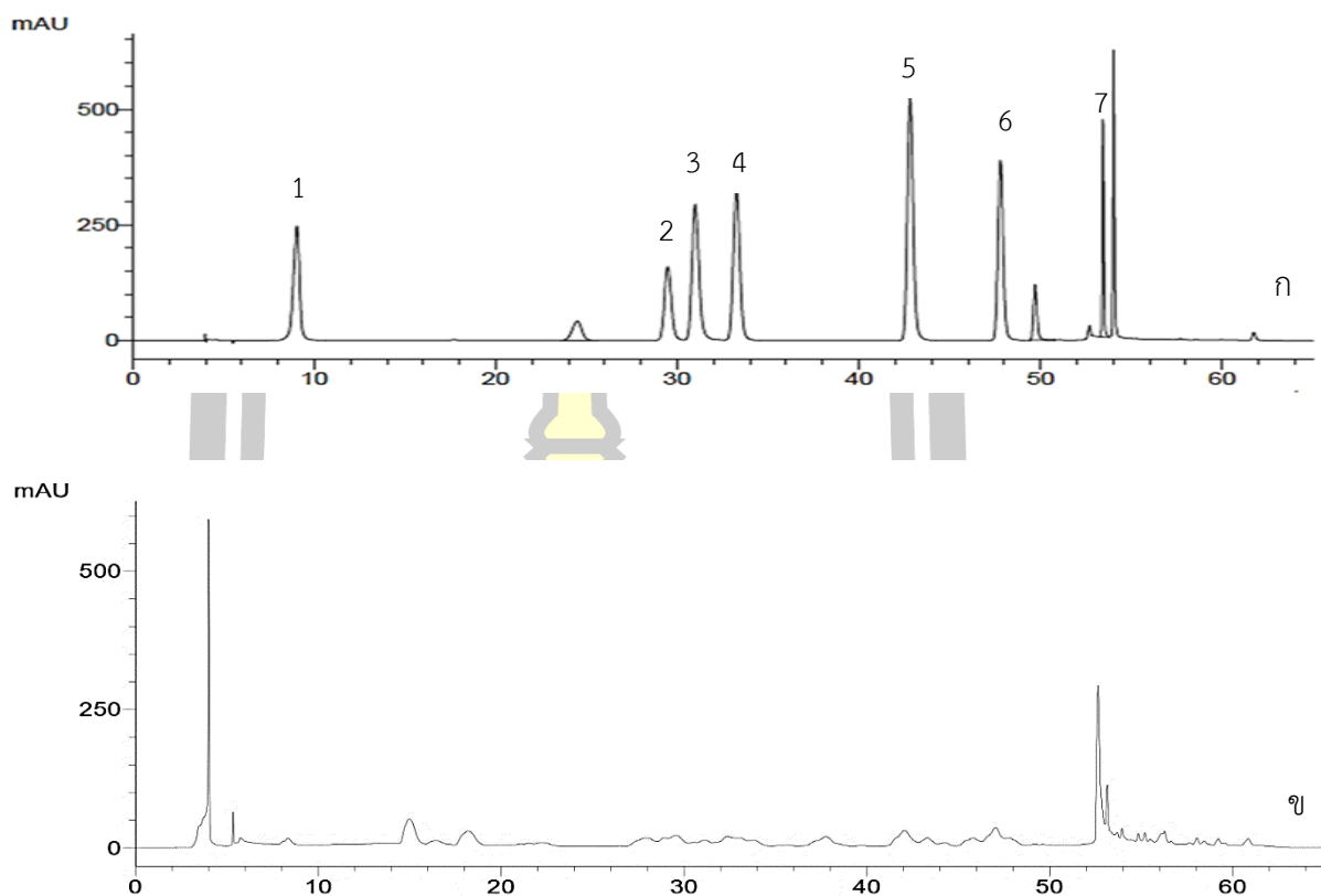
ภาพที่ 12 โครมาโทแกรมแสดงค่าเวลาคงค้างของเปราะโคราชที่เพาะเลี้ยงในหลอดทดลองบนอาหารสูตร MS ที่ไม่เติมฮอร์โมน
