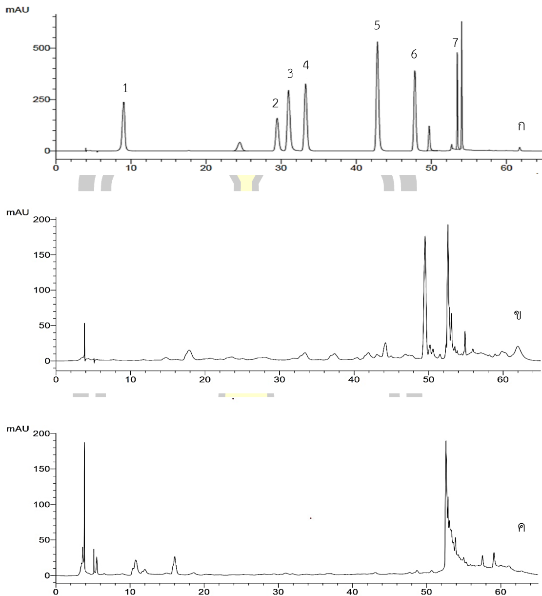
ภาพที่ 11 โครมาโทแกรมแสดงค่าเวลาคงค้างของเปราะโคราชที่เจริญเติบโตในสภาพธรรมชาติ
