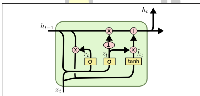
รูปที่ 9 กระบวนการทำงานของ GRU ที่มา: [71]
