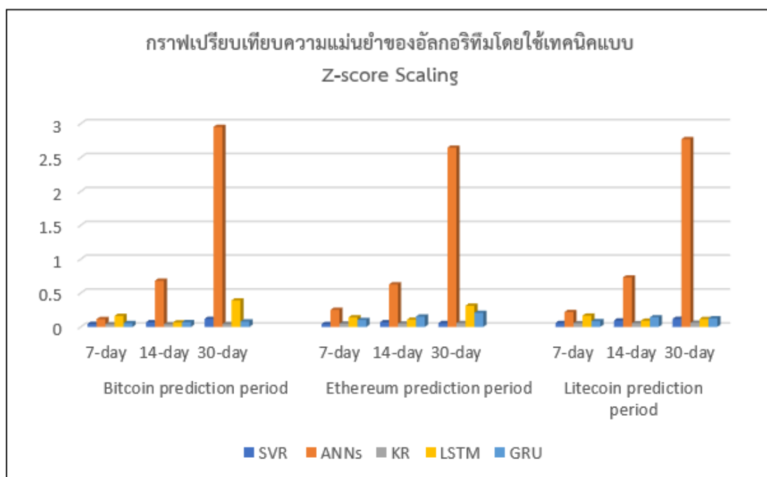
รูปที่ 19 กราฟเปรียบเทียบความแม่นยำของอัลกอริทึมโดยใช้เทคนิคแบบ Z-score Scaling
