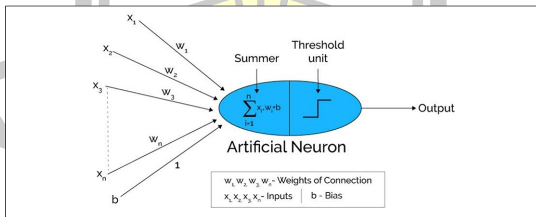
รูปที่ 7 ขั้นตอนการทำงานของ ANNs ที่มา: [62]
