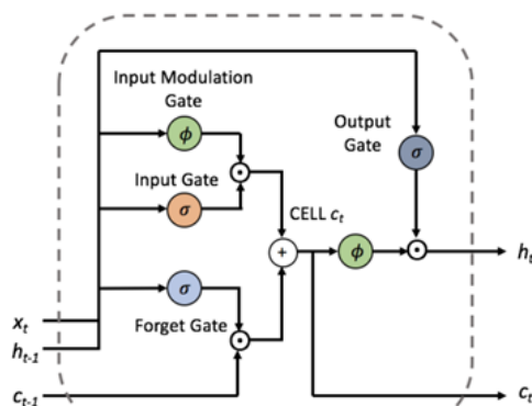
รูปที่ 8 กระบวนการทำงานของ LSTM ที่มา: [65]
